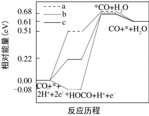
(a) \text{CO}_2 电还原为CO
